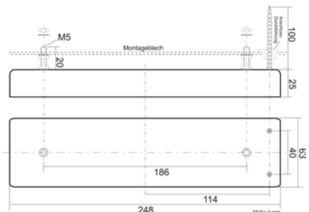
Maßbild Quarzstrahler
