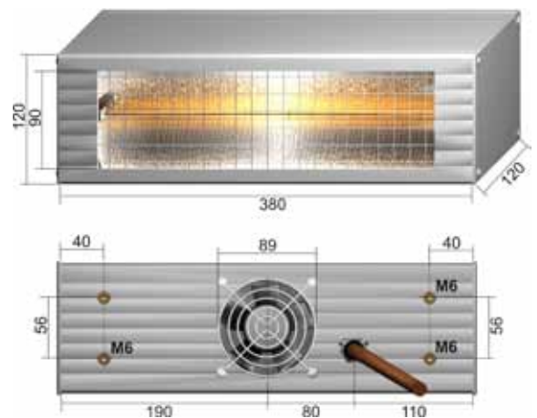
Halogenstrahler IRE 380
